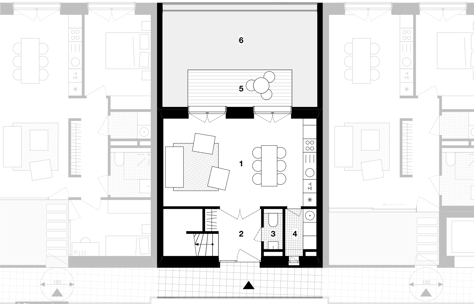
2.Obergeschoss
